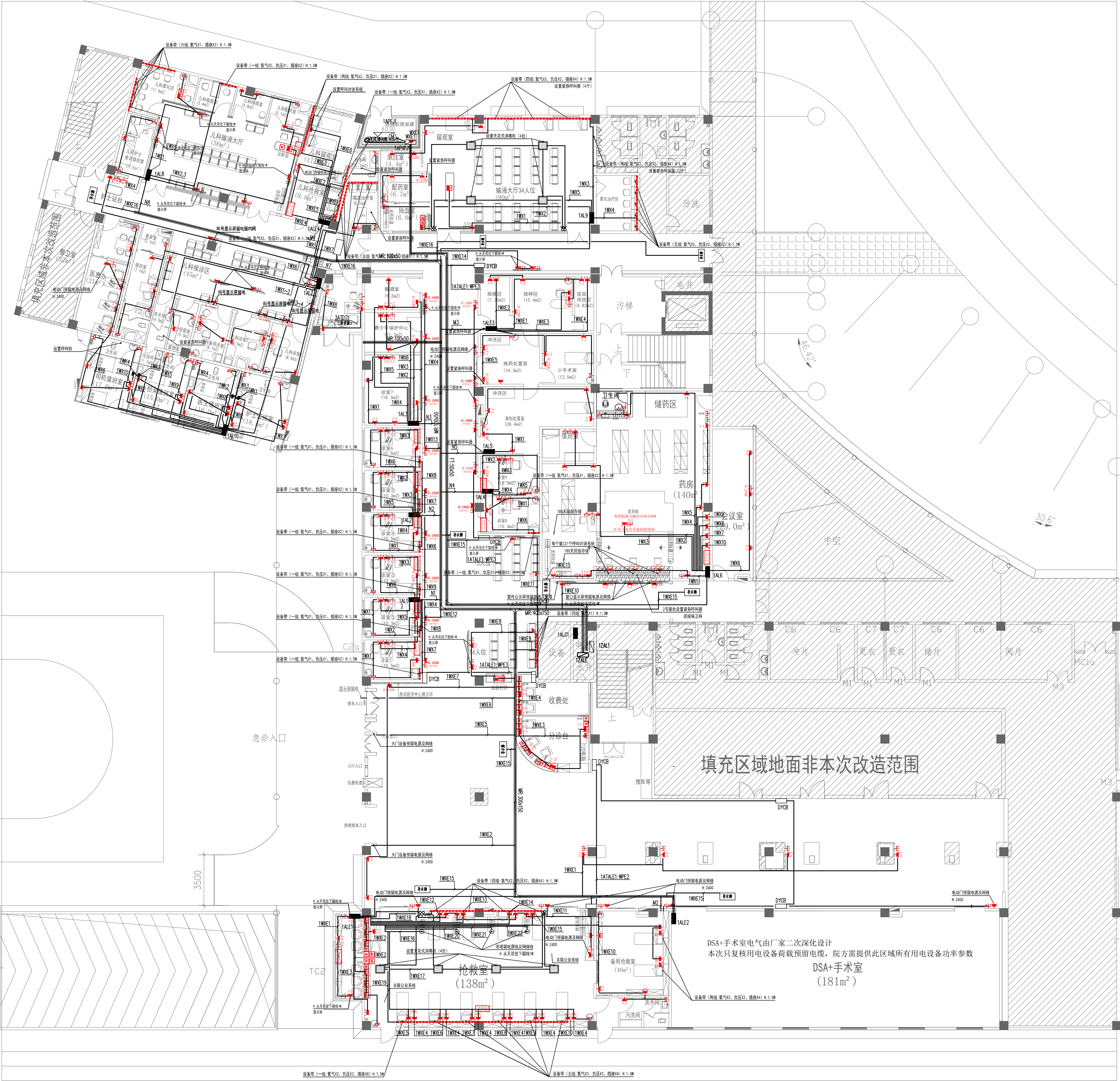
医技急诊楼首层插座配电平面图 1:150
